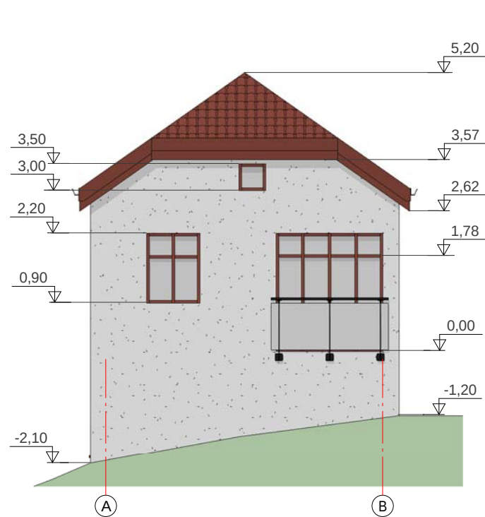
FASADAS TARP AŠIŲ A-B (SPALVINIS SPRENDIMAS)
