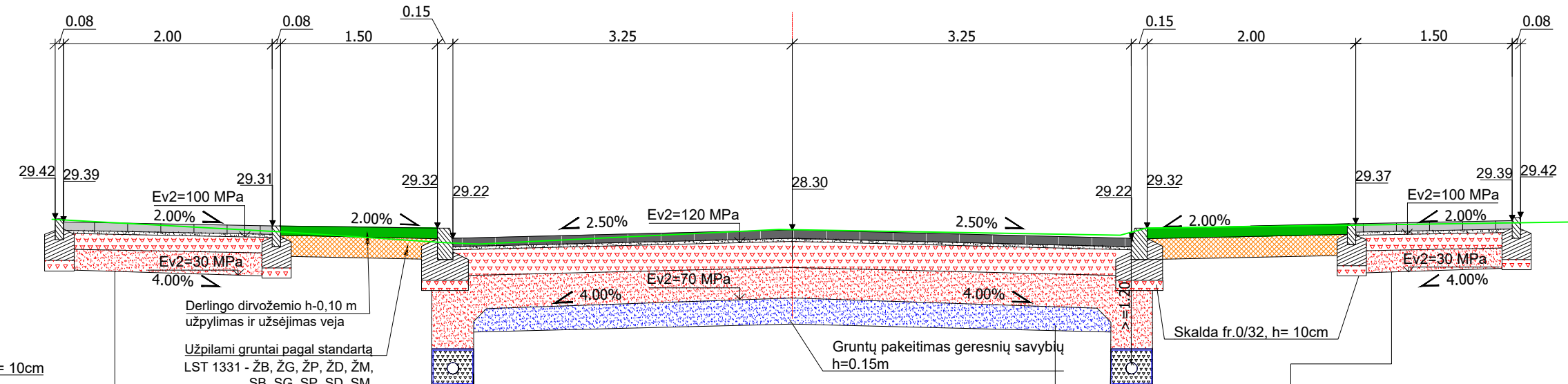
Skersinis profilis 8 PK4+95 D kategorijos gatvė
