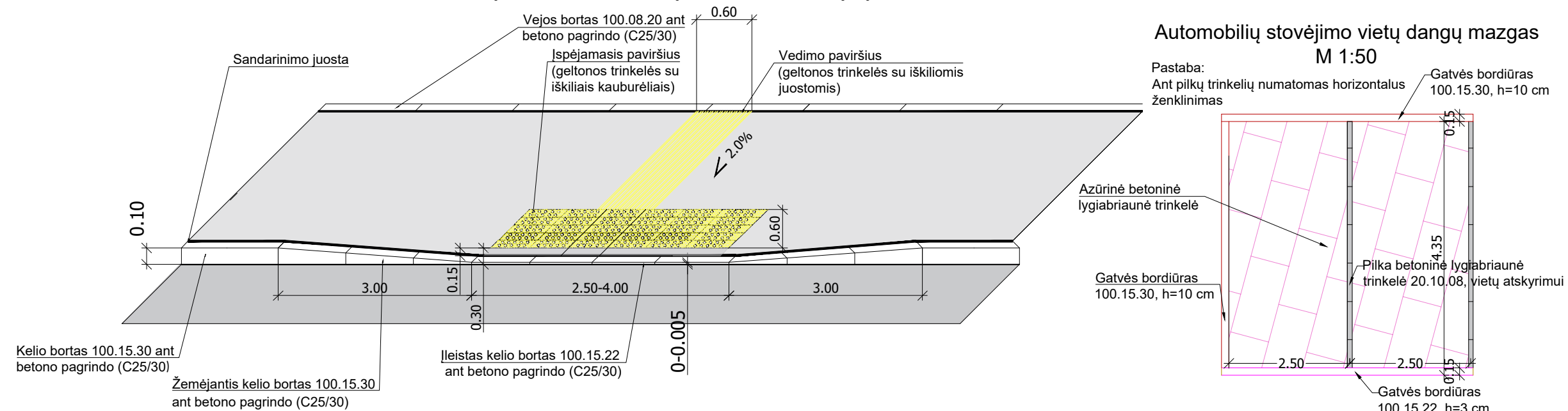
NEREGIŲ VEDIMO SISTEMŲ DETALĖ PĖSČIŲJŲ PERĖJOJE
