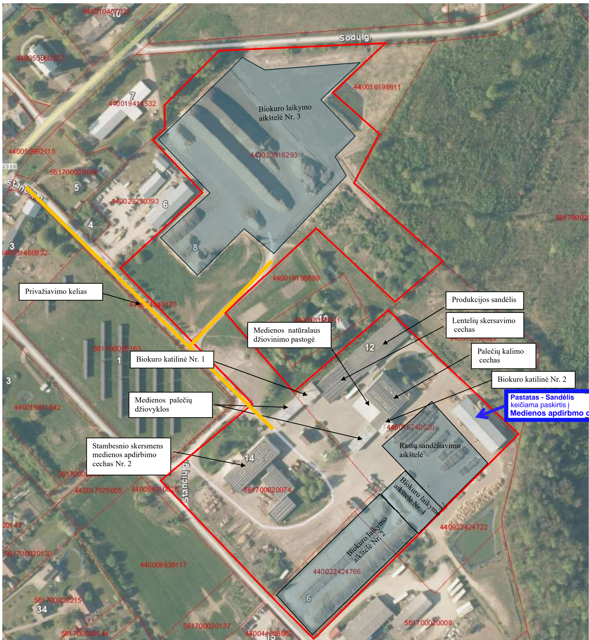
UAB „Babruna“ teritorijos esamų pastatų ir įrenginių planas
