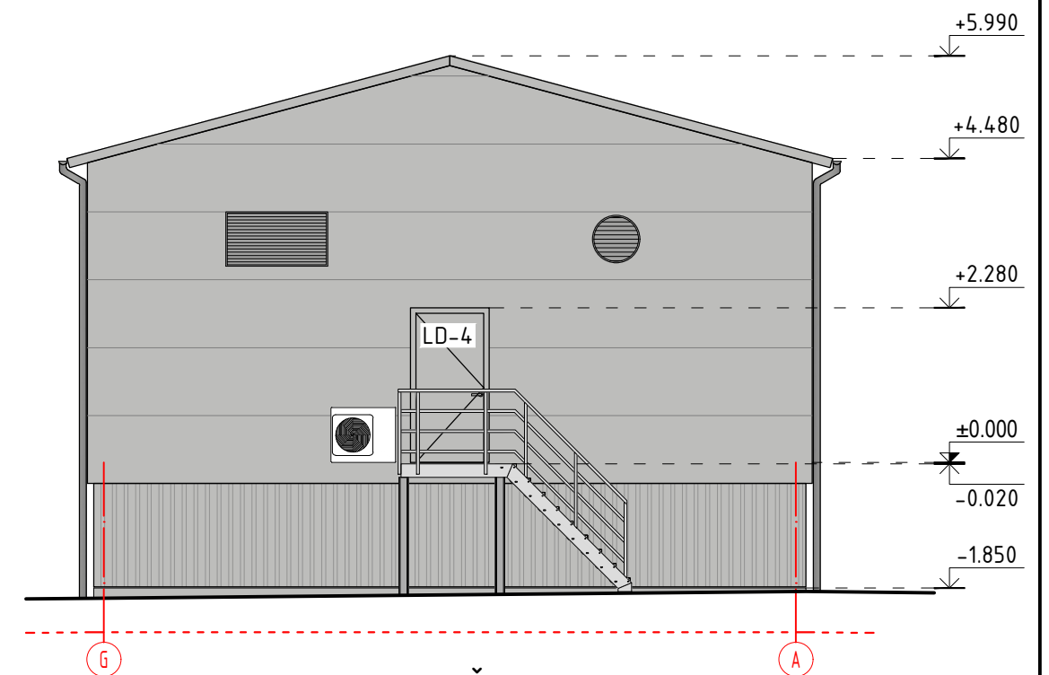
FASADAS TARP AŠIŲ G-A M 1:100
