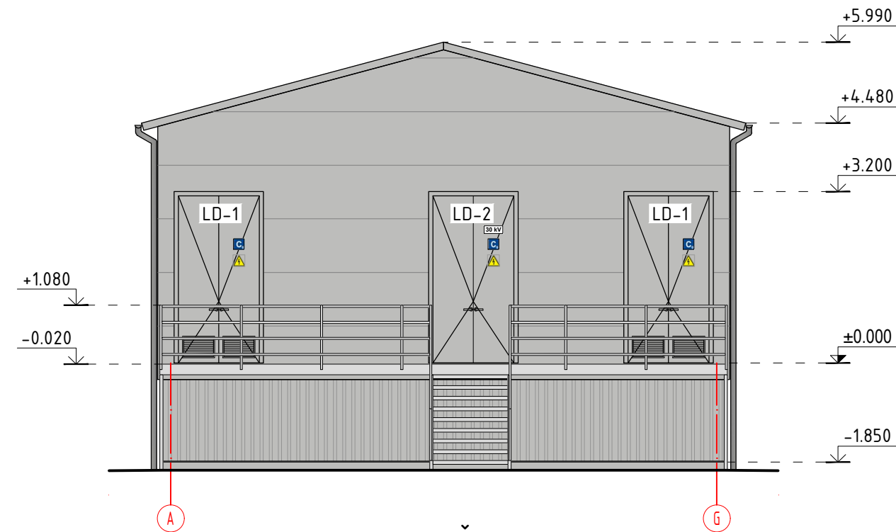
FASADAS TARP AŠIŲ A-G M 1:100
