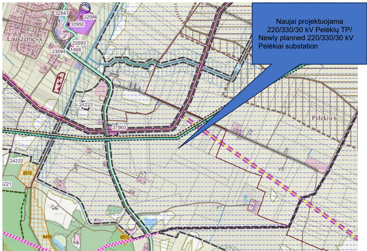
3 pav. Planuojamo statyti statinio schema inžinerinės infrastruktūros vystymo plano kontekste Fig. 3. Schematic diagram of the planned structure in the context of the engineering infrastructure development plan
